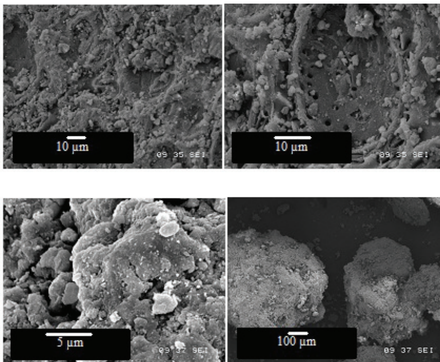
Figura 4. Microscopia obtenida en SEM del mineral limonita
