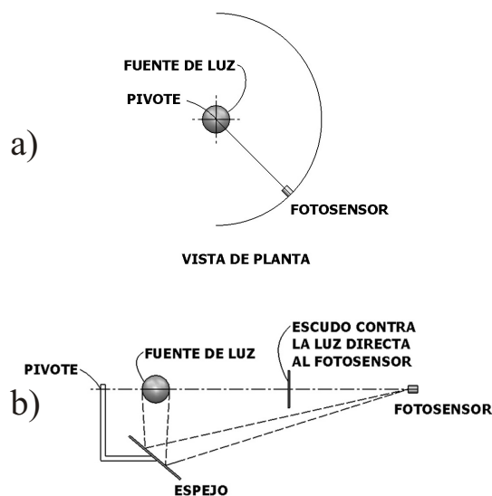
Figura 4. Diferentes principios de funcionamiento de fotogoniómetros tipo C. (Adaptado de IES Lighting Handbook, 1987, Illuminating Engineering Society of North America).
