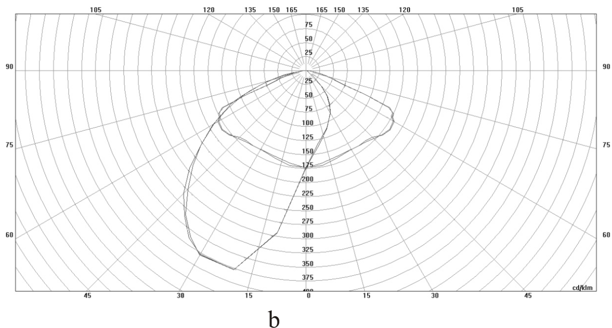
Figura 11. Repetibilidad. a) Valores de iluminancia horizontal (luxes) sobre una calzada de 10m x 36 m, obtenidos en dos mediciones consecutivas utilizando el fotogoniómetro construido en este proyecto. Vista superior. Luminarias a escala 1:250 ubicadas en las esquinas inferiores. b) diagramas polares (cd/klm) de luminarias (referencia Amazonas), obtenidos en 2 mediciones consecutivas y utilizando el fotogoniómetro construido en este proyecto.
