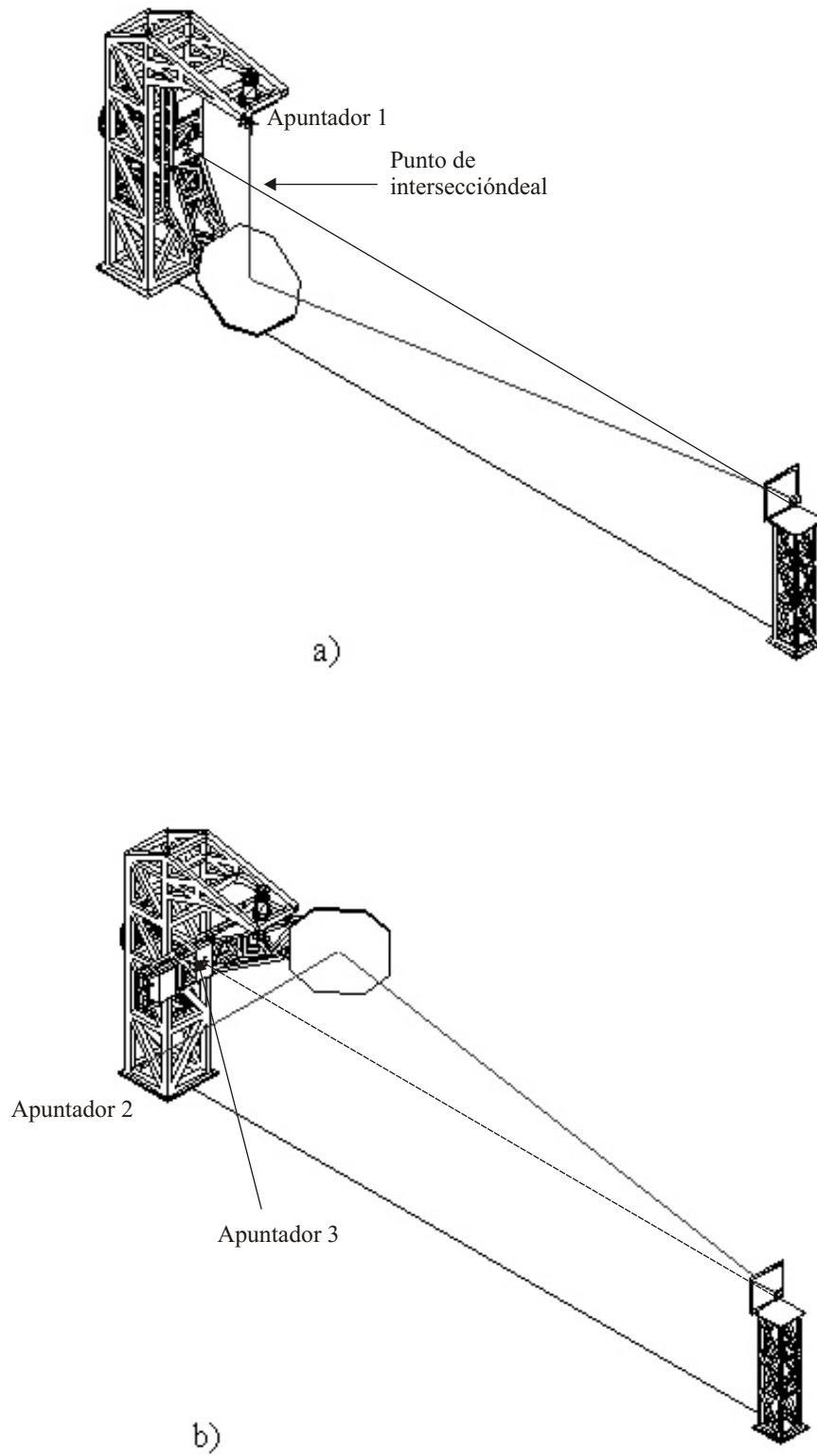
Figura 10. Representación de la metodología de calibración y verificación realizada utilizando apuntadores láser. a) brazo colocado a 90^\circ , b) brazo colocado a 180^\circ .
