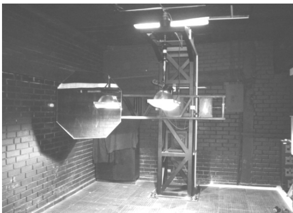
Figura 9. Fotogoniómetro construido y calibrado en el laboratorio de fotometrías de Roy Alpha S.A. con luminaria bajo prueba.
