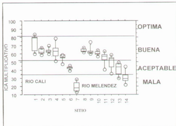
Gráfico 21. Ríos Cali y Meléndez. Índice (Multiplicativo) de calidad (NSF) para los distintos sitios de muestreo.
