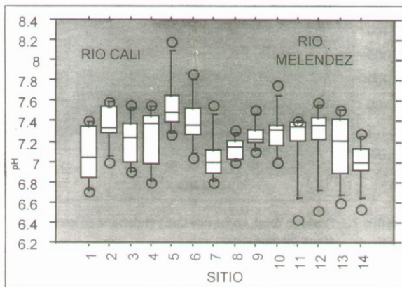
Gráfico 9. Distribución del pH en los ríos Cali y Meléndez, en los distintos sitios de muestreo.
