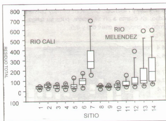
Gráfico 7. Residuo Total, en los ríos Cali y Meléndez en los distintos sitios de muestreo
