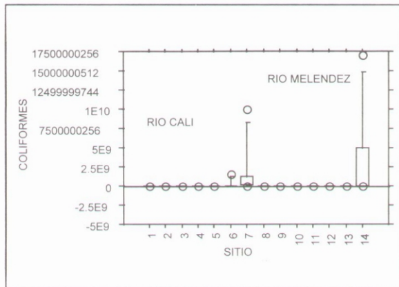
Gráfico 18. Coliformes fecales en los distintos sitios de muestreo de los ríos Cali y Meléndez
