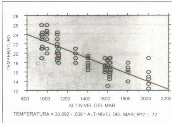
Gráfico 17. Asociación entre la temperatura del agua y la altura sobre el nivel del mar
