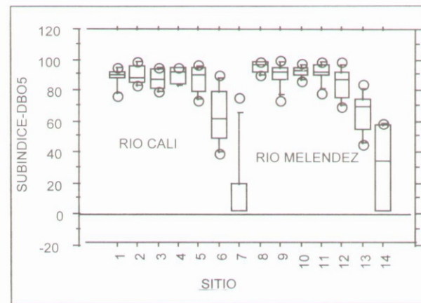
Gráfico 4. Subíndice de Calidad, con respecto a la DBO 5 (NSF), la escala es de 0 a 100 (Óptimo).
