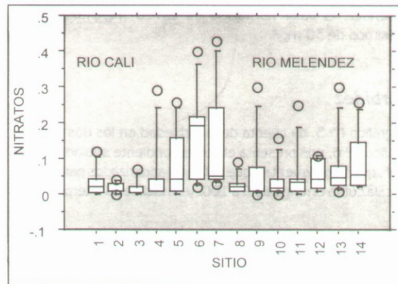
Gráfico 11. Distribución del parámetro Nitratos, en los distintos sitios de muestreo de los ríos Cali y Meléndez
