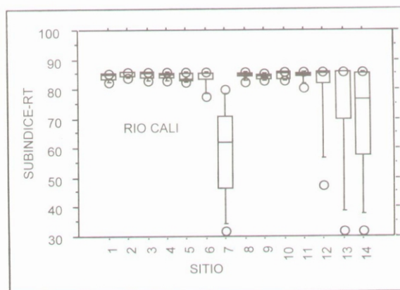
Gráfico 8. Subíndice de calidad, con respecto al Residuo Total, en los ríos Cali y Meléndez en los distintos sitios de muestreo. La escala es de 0 a 100.
