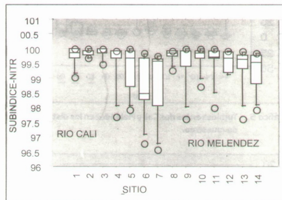
Gráfico 12. Subíndice de la NSF, para Nitratos, en los distintos sitios de muestreo de los ríos Cali y Meléndez.
