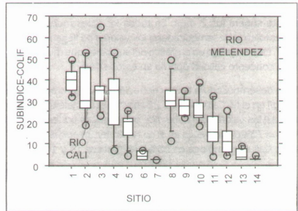
Gráfico 19. Subíndice NSF, para coliformes fecales en los distintos sitios de muestreo de los ríos Cali y Meléndez
