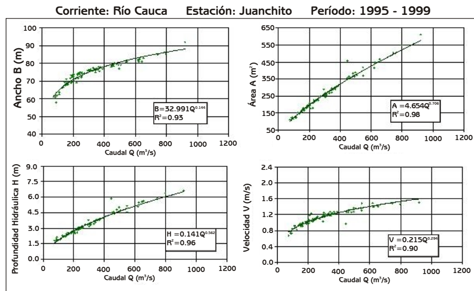
Figura No. 1 - Relaciones Caudal vs. Parámetros Hidráulicos y Geométricos
