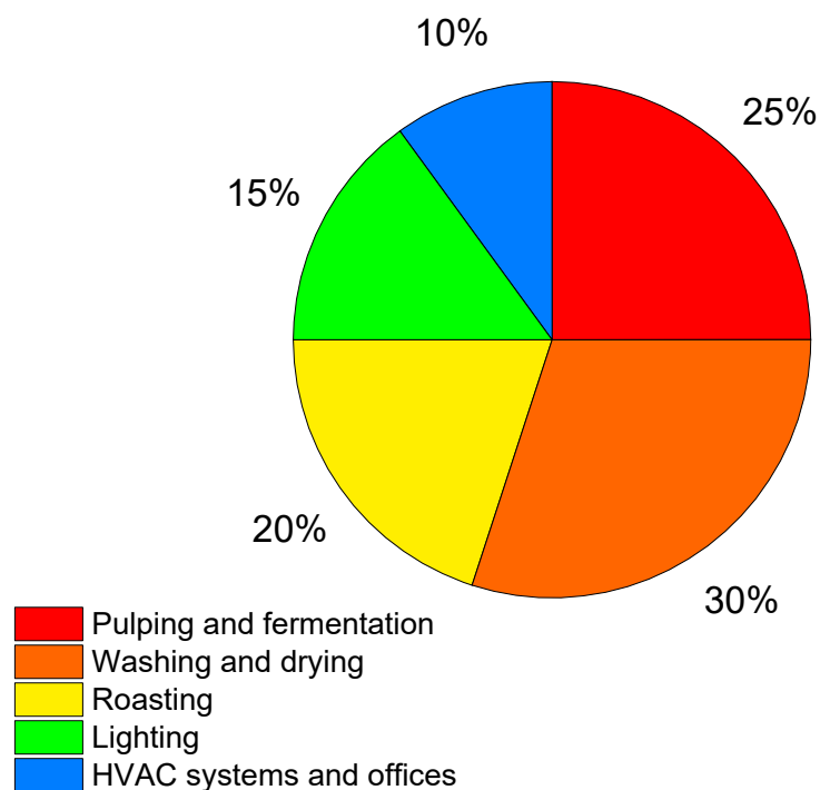
Figura 5. Distribución porcentual del consumo eléctrico por área en 2023
