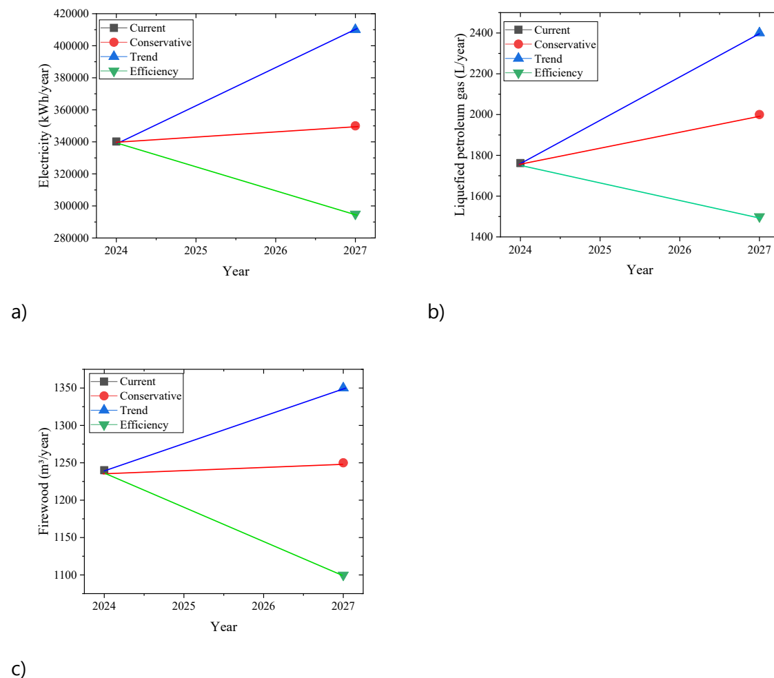
Figura 6. Proyecciones de consumo energético en tres escenarios para el periodo 2024–2027: (a) electricidad (kWh/año), (b) gas licuado de petróleo (L/año) y (c) leña (m 3 /año). El escenario de tendencia indica un aumento esperado de la demanda energética, especialmente debido a procesos térmicos y mecánicos, mientras que el escenario de eficiencia sugiere una reducción progresiva asociada a la implementación de medidas sistemáticas de gestión energética alineadas con la ISO 50001.
