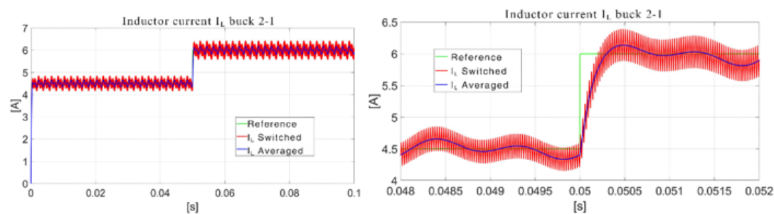
Figura 14. Comparación de la corriente a través del inductor para el modo de funcionamiento Buck2-1 (modelo de circuito convertidor conmutado vs. modelo de circuito canonica promediado y linealizado)
