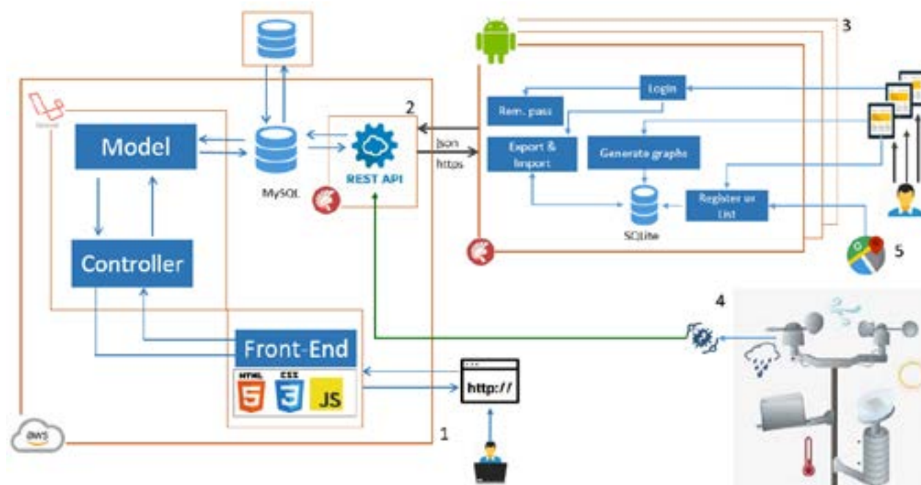
Figura 4. Arquitectura SARA
