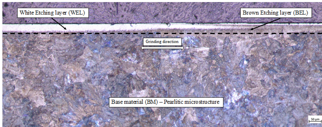
Figura 5. Vista transversal de la microestructura tras el proceso de rectificado. Vista longitudinal
