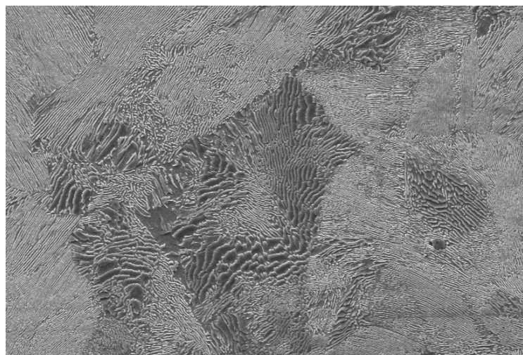
Figura 1. Microestructura del material ferroviario R260. SEM. (2000x). Acero perlítico.
