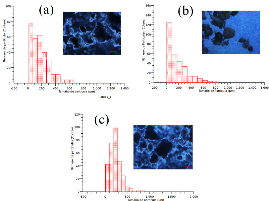
Figura 2. (a) tamaño de partícula en microscopía óptica; CFC1 x10 escala 100 µm, (b) CFC2 x10 escala 100 µm, (c) CFC3 x10 escala 100 µm. Fuente: autores
