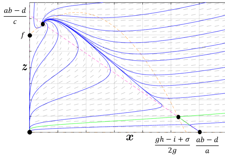
Figura 2. Plano fase para el caso 2. Figura del autor.
