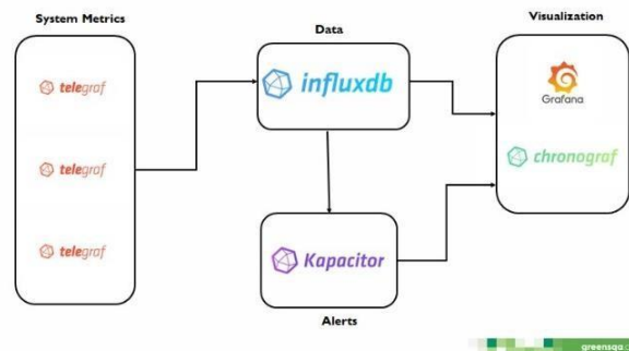
Figura 2. Arquitectura pila TICK con Grafana.
