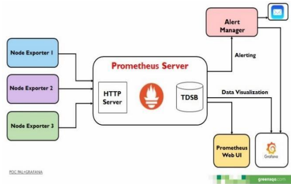
Figura 1. Arquitectura pila PALG. Fuente: propia
